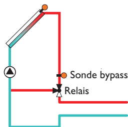
variante vanne:
