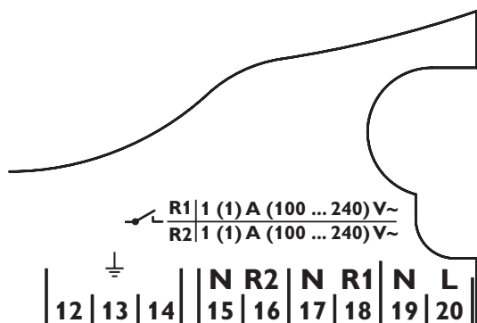
bornes de terre et bornes pour appareils électriques
