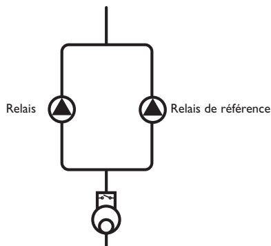
Exemple schématique de pompes doubles avec un débitmètre en amont
