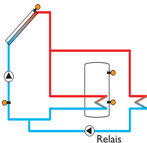
Variante pompe
