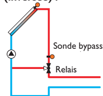
Variante vanne (inversée):
