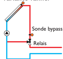
Variante vanne:
