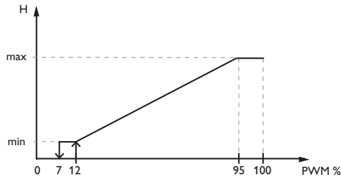
Courbe de commande : PWM; courbe : Chauffage
