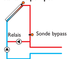
Variante pompe:
